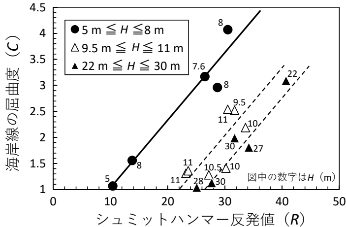
第5図 海岸線の屈曲度 (C) に与える縄文海進以降の離水量 (H) の影響
