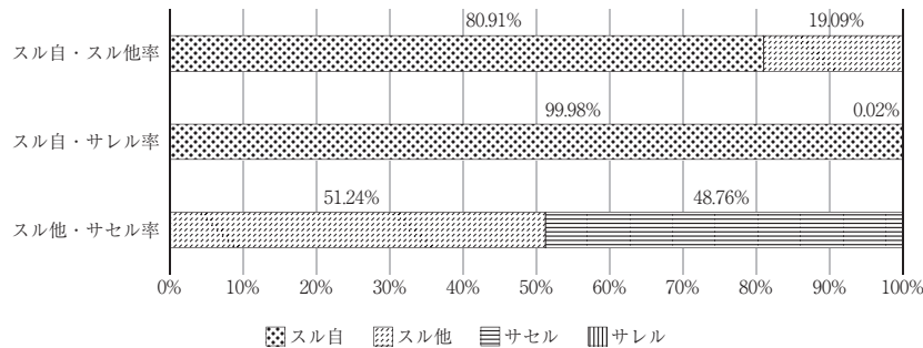
図5 「オープン」の各形式の使用率
