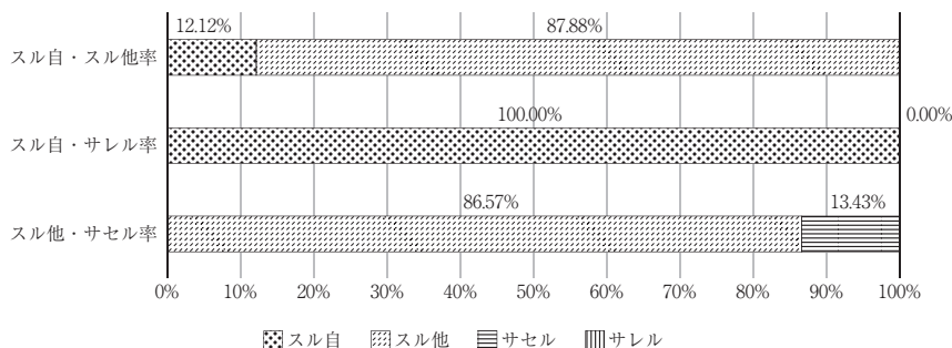
図13 「チェンジ」の各形式の使用率
