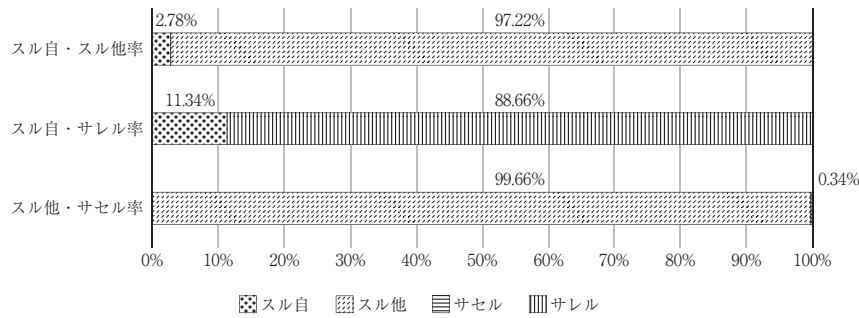
図20 「カット」の各形式の使用率
