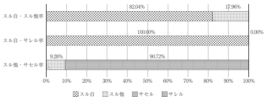
図18 「リラックス」の各形式の使用率
