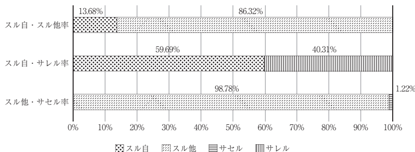
図22 「ノック」の各形式の使用率
