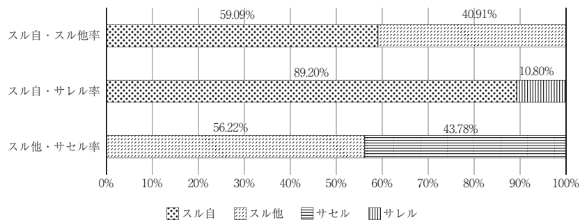
図2 「アップ」の各形式の使用率
