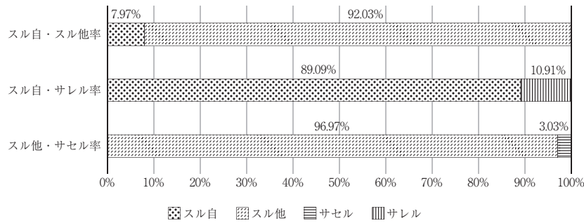
図19 「チェック」の各形式の使用率
