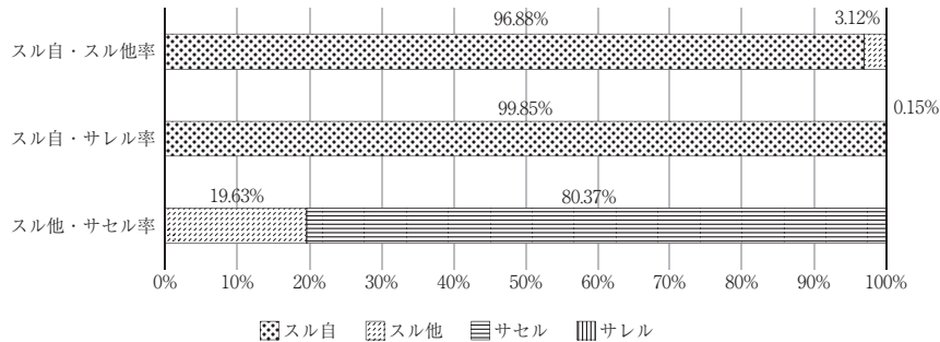
図3 「ダウン」の各形式の使用率
