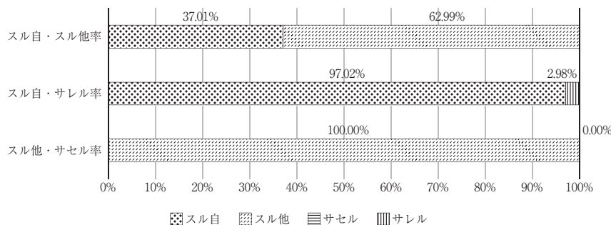
図23 「インタビュー」の各形式の使用率
