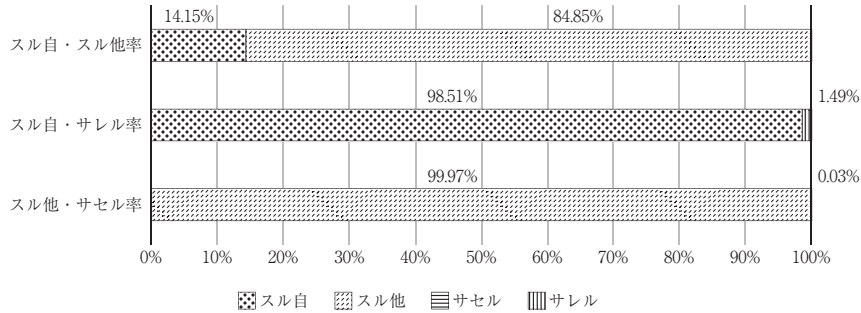
図15 「リード」の各形式の使用率
