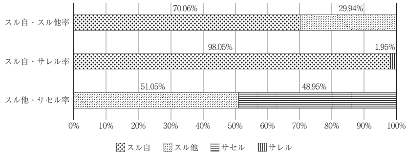
図8 「ストップ」の各形式の使用率
