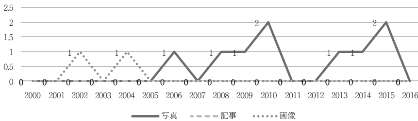
図11 「聞蔵Ⅱ」における「アップロードする」の経年変化
