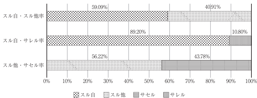
図9 「アップ」の各形式の使用率
