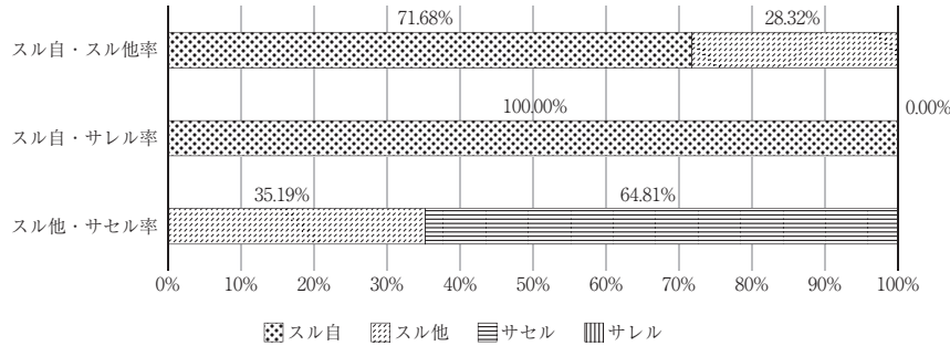
図17 「スタート」の各形式の使用率
