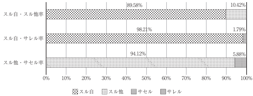
図4 「サイン」の各形式の使用率
