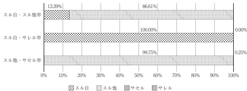
図14 「オーバー」の各形式の使用率
