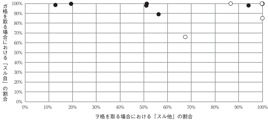
図24 外来語サ変動詞がガ格ヲ格それぞれを取る場合における「スル」の使用率
