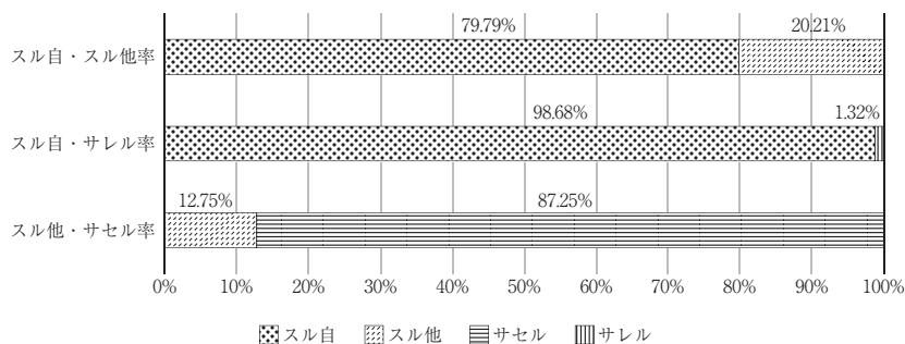
図6 「スライド」の各形式の使用率
