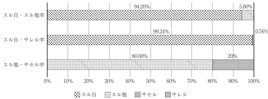
図21 「チャレンジ」の各形式の使用率
