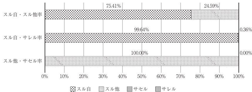
図7 「コメント」の各形式の使用率
