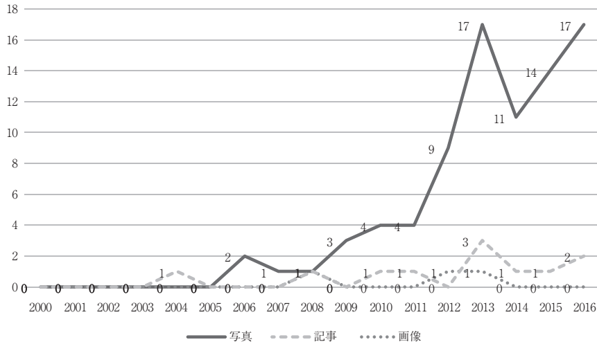
図10 「聞蔵Ⅱ」における「アップする」の経年変化
