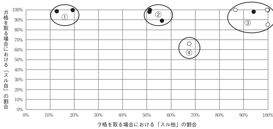
図25 外来語サ変動詞がガ格・ヲ格をそれぞれに取る場合の「スル」の使用率
