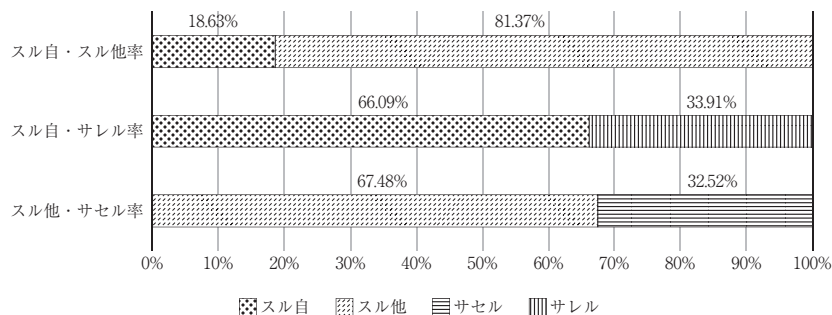
図16 「リフレッシュ」の各形式の使用率
