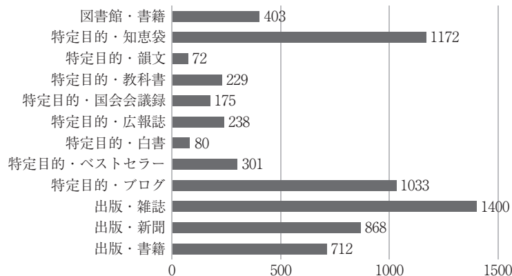
図1 外来語サ変動詞の各ジャンルにおける出現頻度 (数値はPMW)
