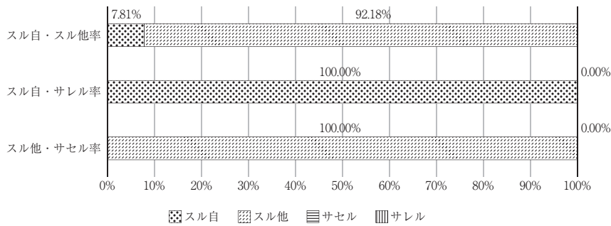
図12 「サービス」の各形式の使用率
